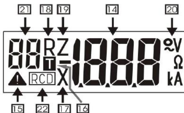
Рисунок 9 - Дисплей прибора MZC-303E
