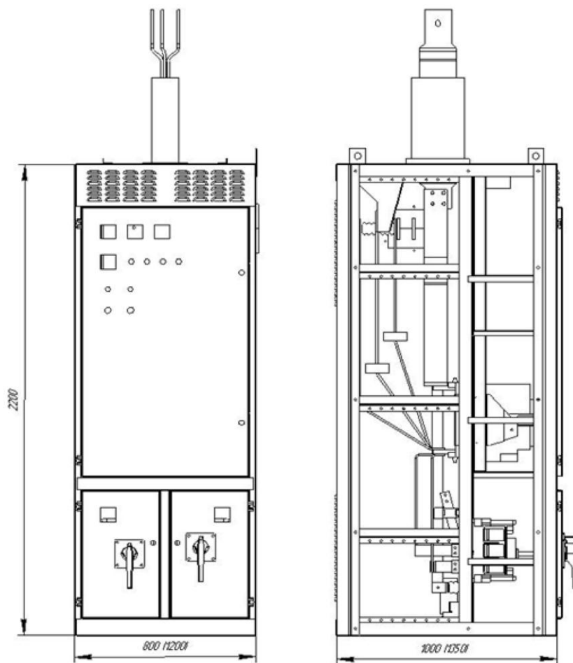
Рисунок 1 - Шкаф ШНВ
