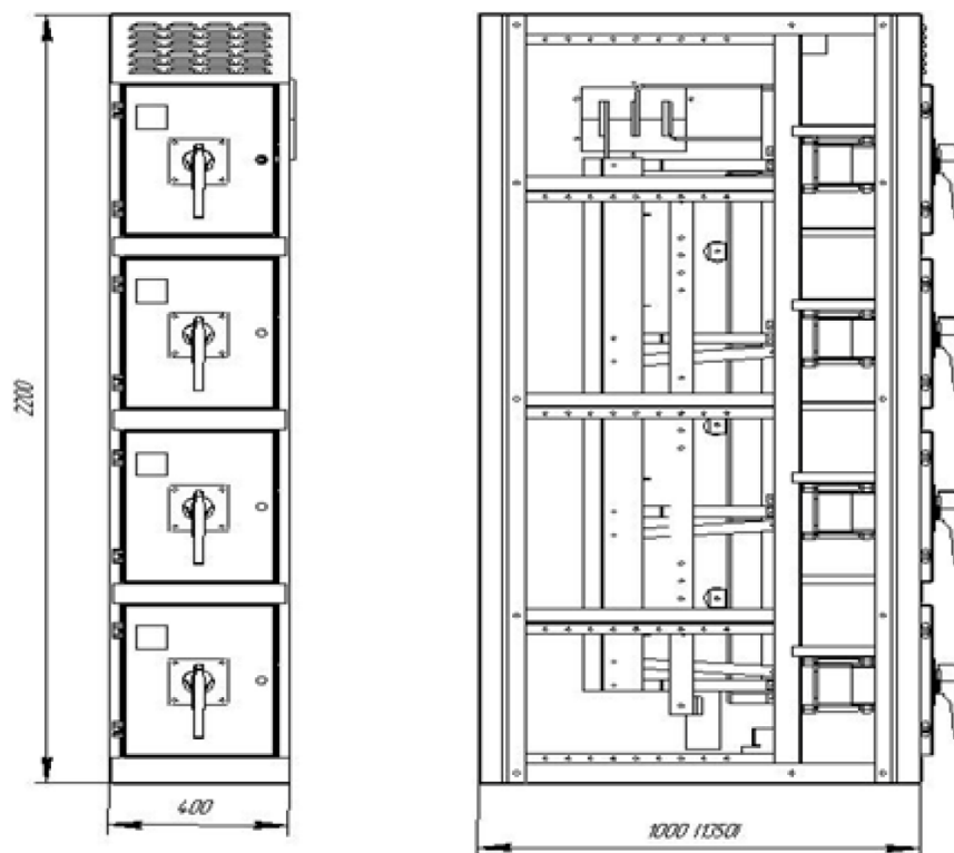
Рисунок 3 - Шкаф ШНЛ шириной 400 мм
