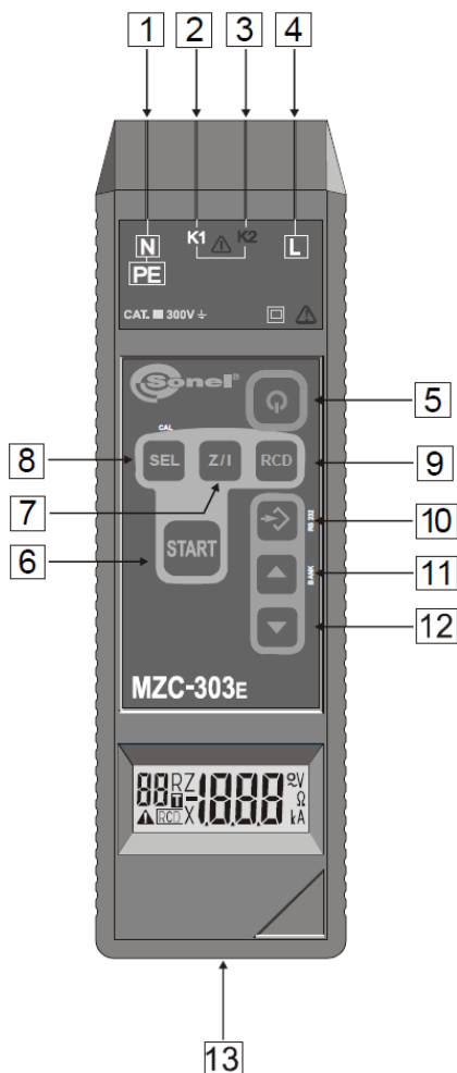
Рисунок 8 – Цифровой прибор MZC-303E:
