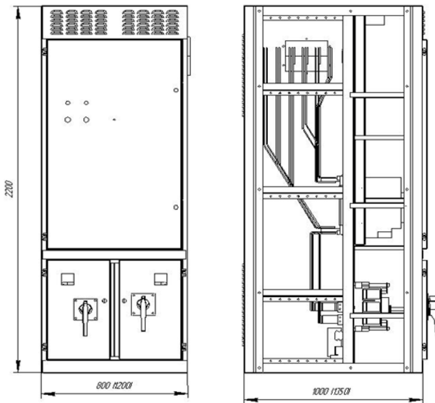
Рисунок 2 - Шкаф ШНС
