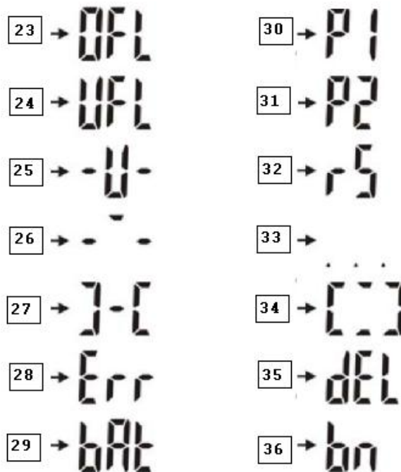
Рисунок 10 - Символы, отображаемые на дисплее прибора MZC-303E
