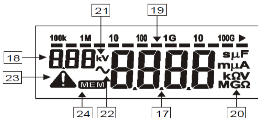
Рисунок 5 - Жидкокристаллический дисплей прибора МІС-2500:
