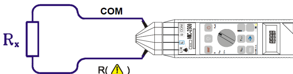
Рисунок 6 - Подключение прибора MIC-2500 при измерении сопротивления изоляции по двухпроводной схеме
